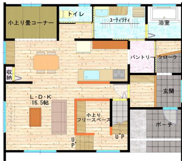
1階平面図
